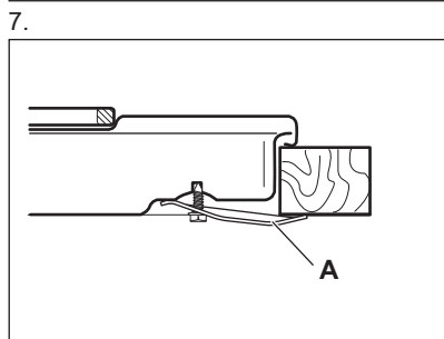
А. Идущая в комплекте крепежная скоба
